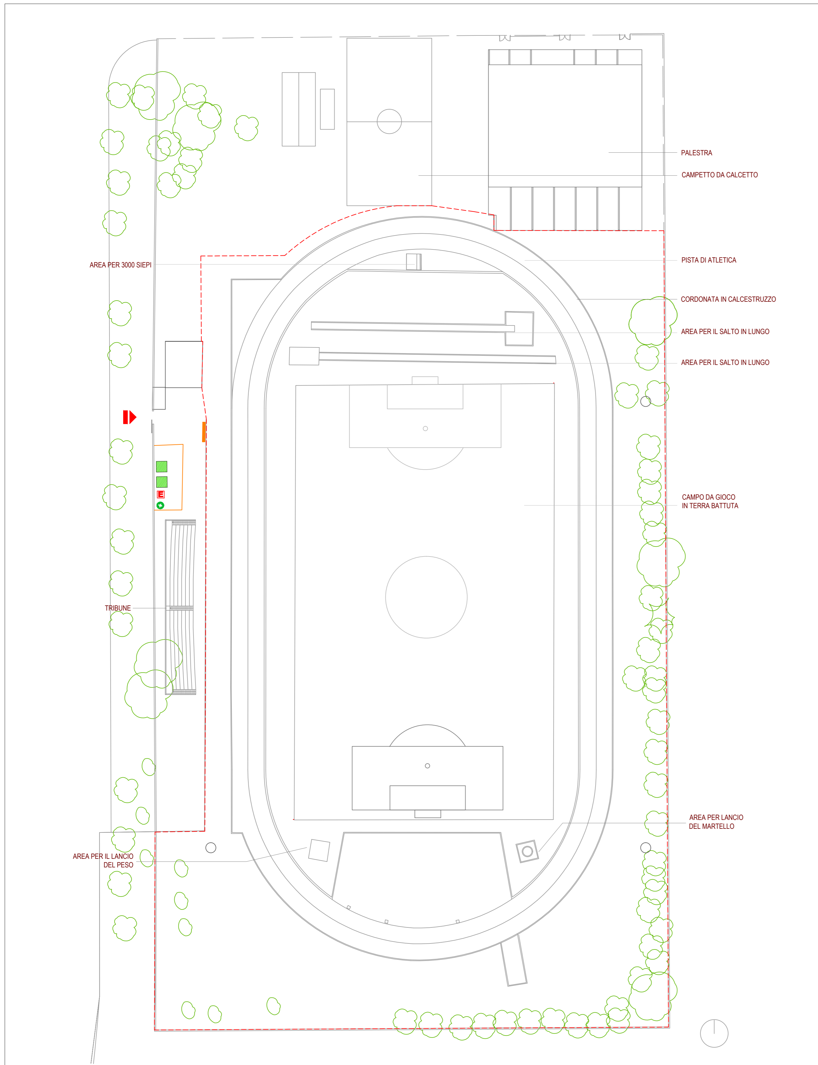
Planimetria di cantiere_Scala 1:500
